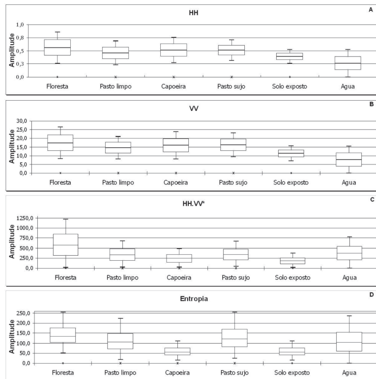
Figura 3 - Gráficos box-plot das classes de uso e cobertura da terra nas imagens TerraSAR em modos A_{HH} (a), A_{VV} (b), A_{<HH,VV*>} (c) e Entropia (d).
