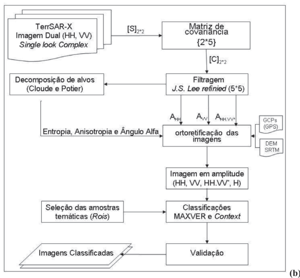
Figura 2 - Diagrama com a organização geral do trabalho (a) e procedimentos adotados nas etapas de pré-processamento e classificação (b).
