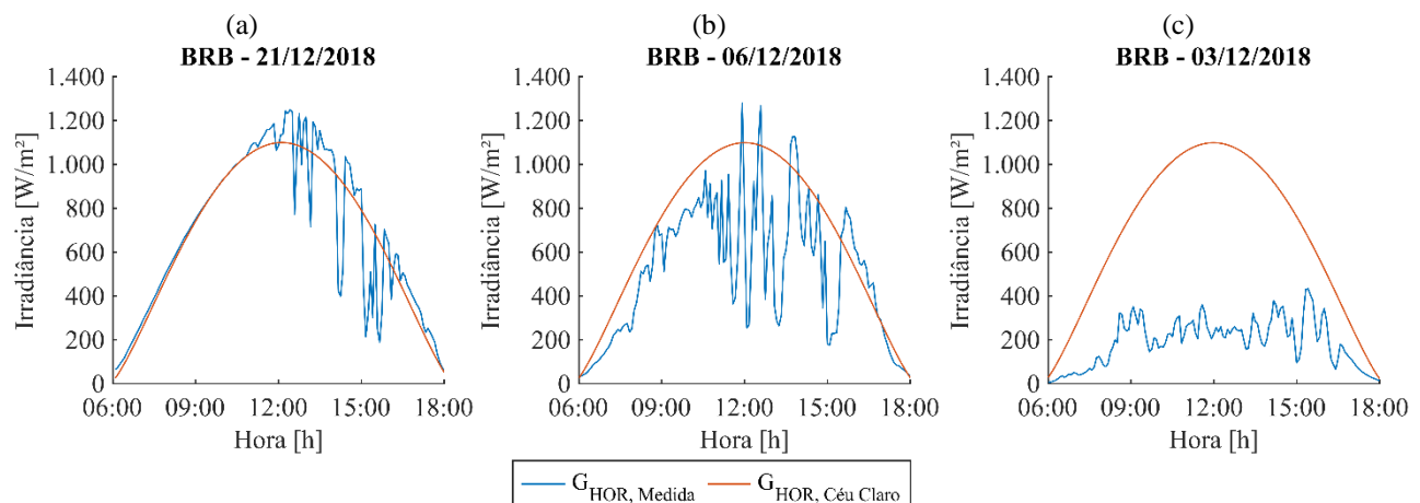
Figura 2 (parte 1 de 2) – Irradiâncias medidas ( G_{HOR,Medida} ) e de céu claro ( G_{HOR,Céu Claro} ) e fotos do céu para: (a) e (d) céu claro, (b) e (e) dia com nuvens esparsas e (c) e (f) dia nublado para três dias de dezembro de 2018 da estação da rede SONDA em Brasília.
