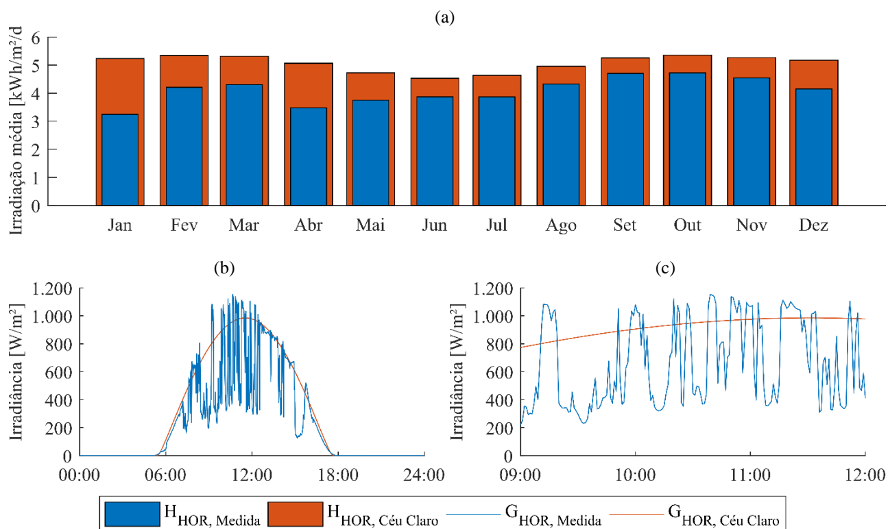
Figura 1 – Variabilidade do recurso solar em escala: (a) irradiação anual (longo prazo), (b) irradiação diária (médio prazo) e (c) irradiação sub-horária (curto prazo).
