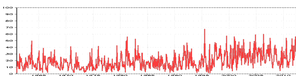
Figura 1 – Área total do Brasil afetada por episódios de seca, com base nos dados de precipitação do período de 1961 a 2012.
