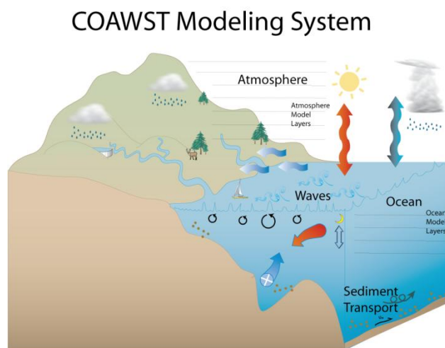
Figura 1. Sistema acoplado Oceano-Atmosfera-Onda-Sedimentos COAWST.
