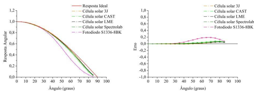
Figura 11 - Curvas médias da resposta angular dos elementos sensores medidos com a fonte de radiação de filamento (esquerda) e curvas médias de erro (direita).
