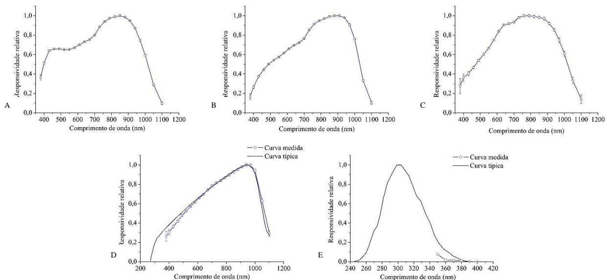
Figura 9 - Curvas da resposta espectral média dos elementos sensores medidos. Células solares Spectrolab (A), CAST (B), LME (C), fotodiodos de Si (D), fotodiodos de TiO 2 (E).
