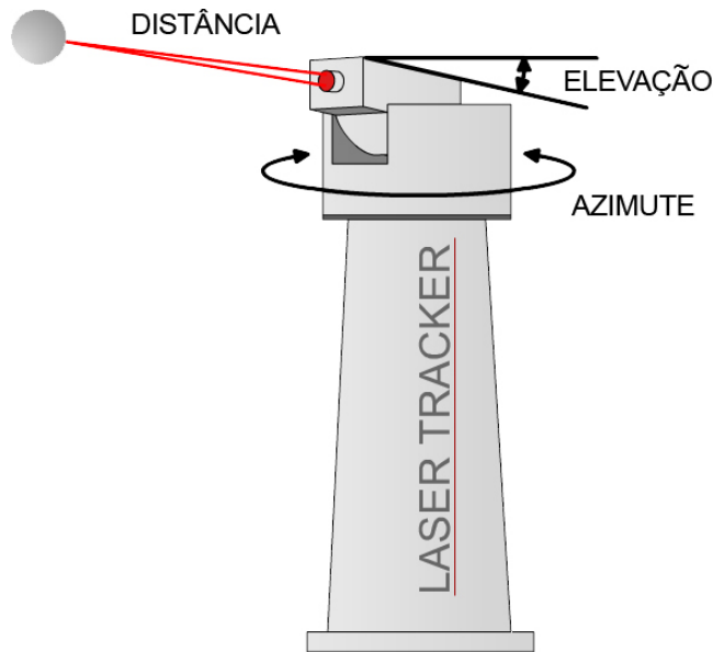
Figura (9). Laser Tracker.
