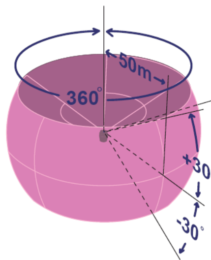
Figura (2). Área de cobertura de um transmissor.
