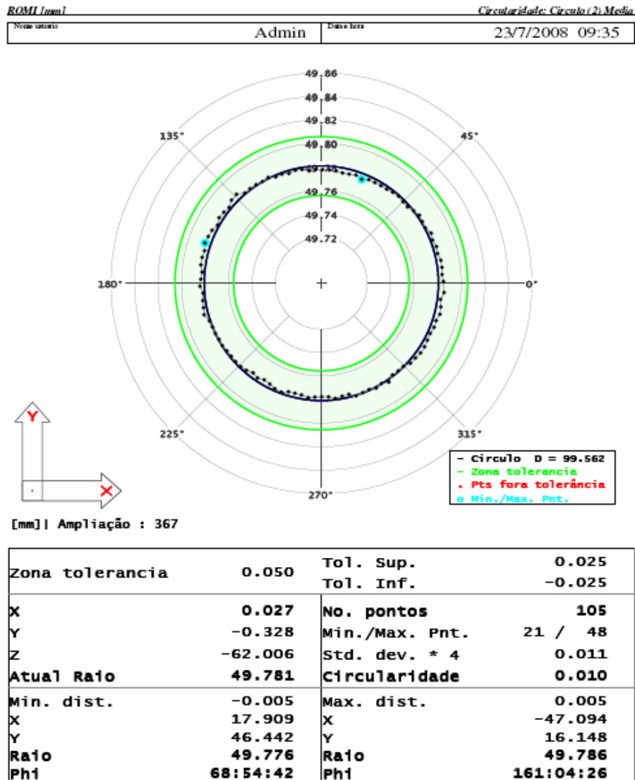
Figura 7: Circularidade do cilindro 2 (maior raio).
