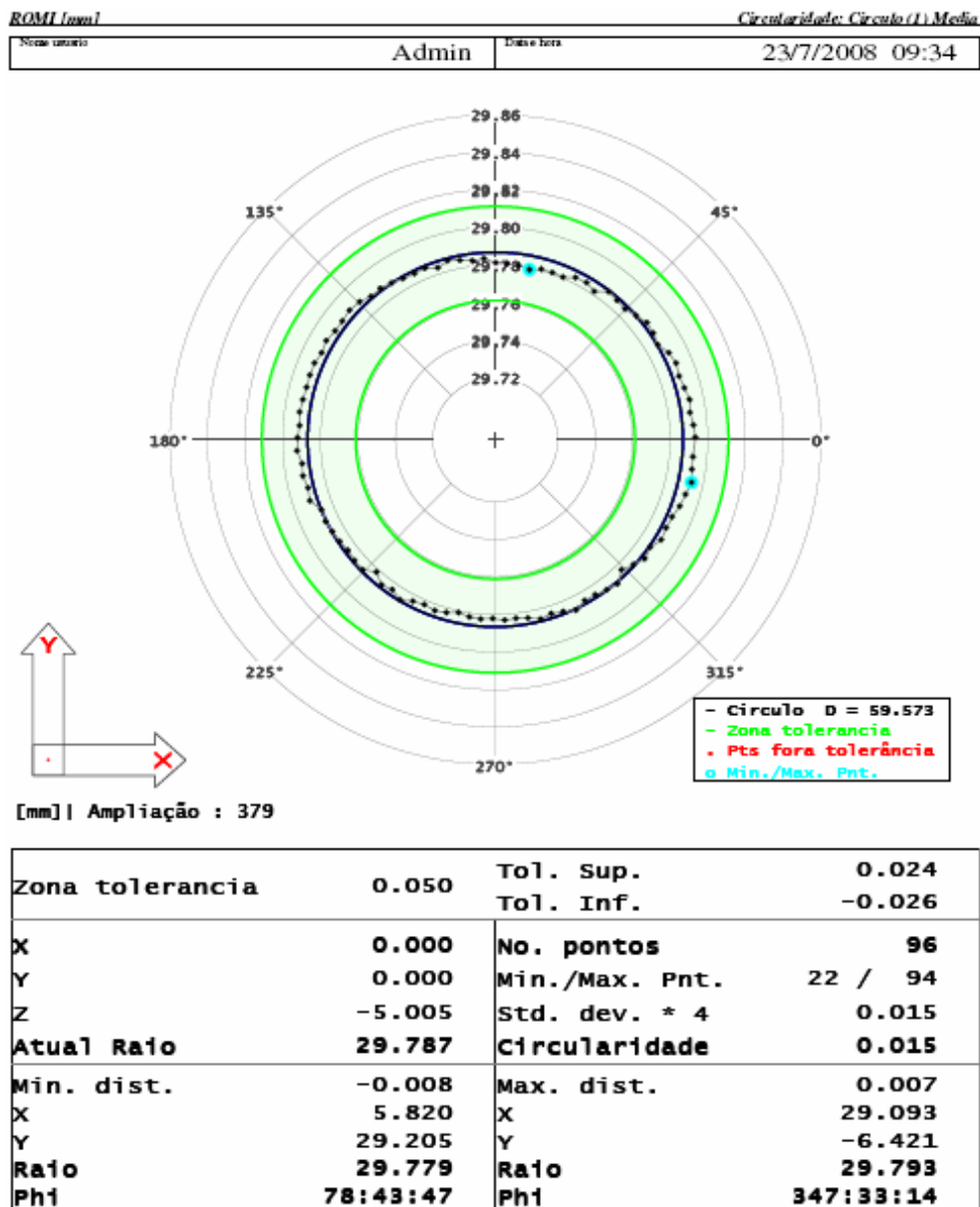
Figura 6: Circularidade do cilindro 1 (menor raio).
