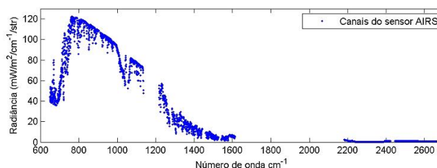
Figura 3 – Espectro simulado de radiação do AIRS.
