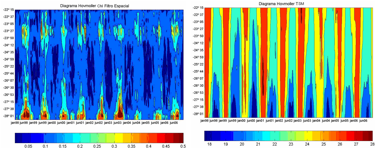
Figura 3 - Diagramas Hovmoller da Chl (na esquerda, em mg.m -3 ) e TSM (na direita, em °C).
