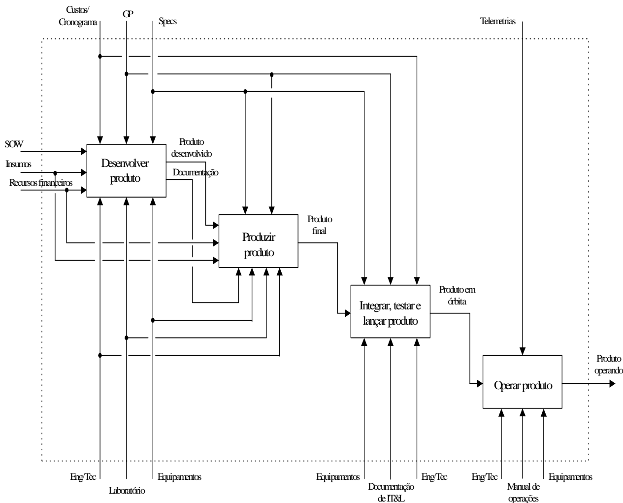
Figura 2. Processos do Ciclo de Vida do TT&C.
