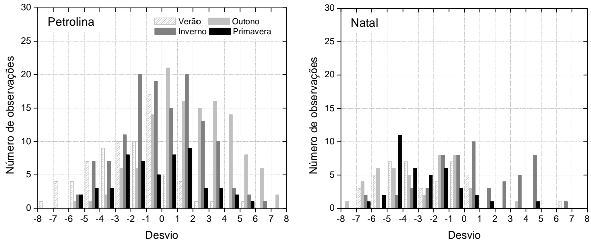
Figura 3 - Histograma sazonal do desvio (satélite - medida).
