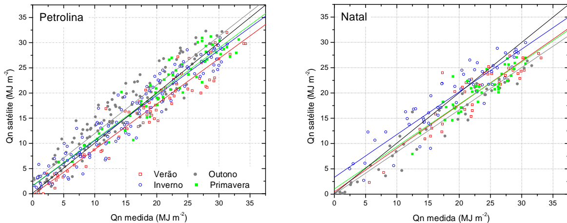
Figura 2 - Irradiação solar direta normal medida e estimada por satélite em distintas épocas do ano. Ajustes lineares entre a Q_n medida e satélite para o verão, outono, inverno e primavera são representados pelas linhas vermelha, cinza, azul e verde, respectivamente.
