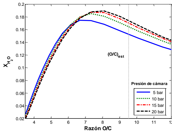
Figura 18. Variación de la fracción molar de H_2O para la reacción N_2O/C_{20}H_{42}/C con porcentaje de masa de 1% de negro de humo.
