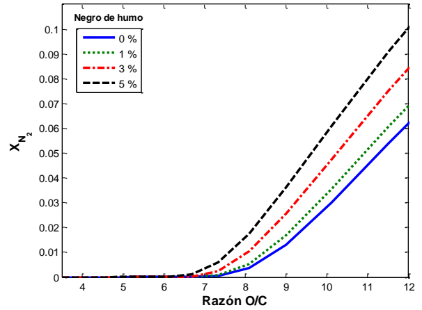
Figura 13. Variación de la fracción molar de N_2 para la reacción N_2O/C_{20}H_{42}/C con presión de cámara de 10 bar.
