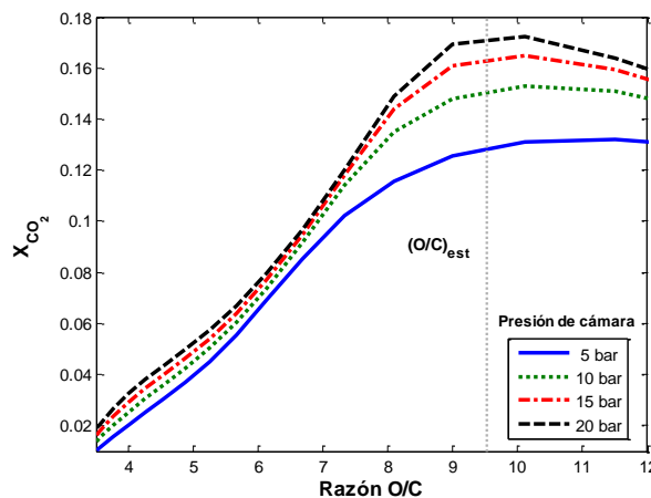
Figura 17. Variación de la fracción molar de CO_2 para la reacción N_2O/C_{20}H_{42}/C con porcentaje de masa de 1% de negro de humo.
