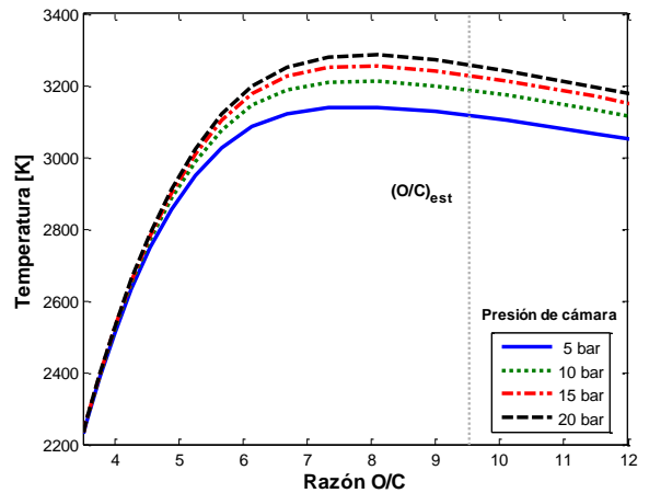
Figura 14. Variación de la temperatura en relación a la razón de O/C para la reacción N_2O/C_{20}H_{42}/C con porcentaje de masa de 1% de negro de humo.
