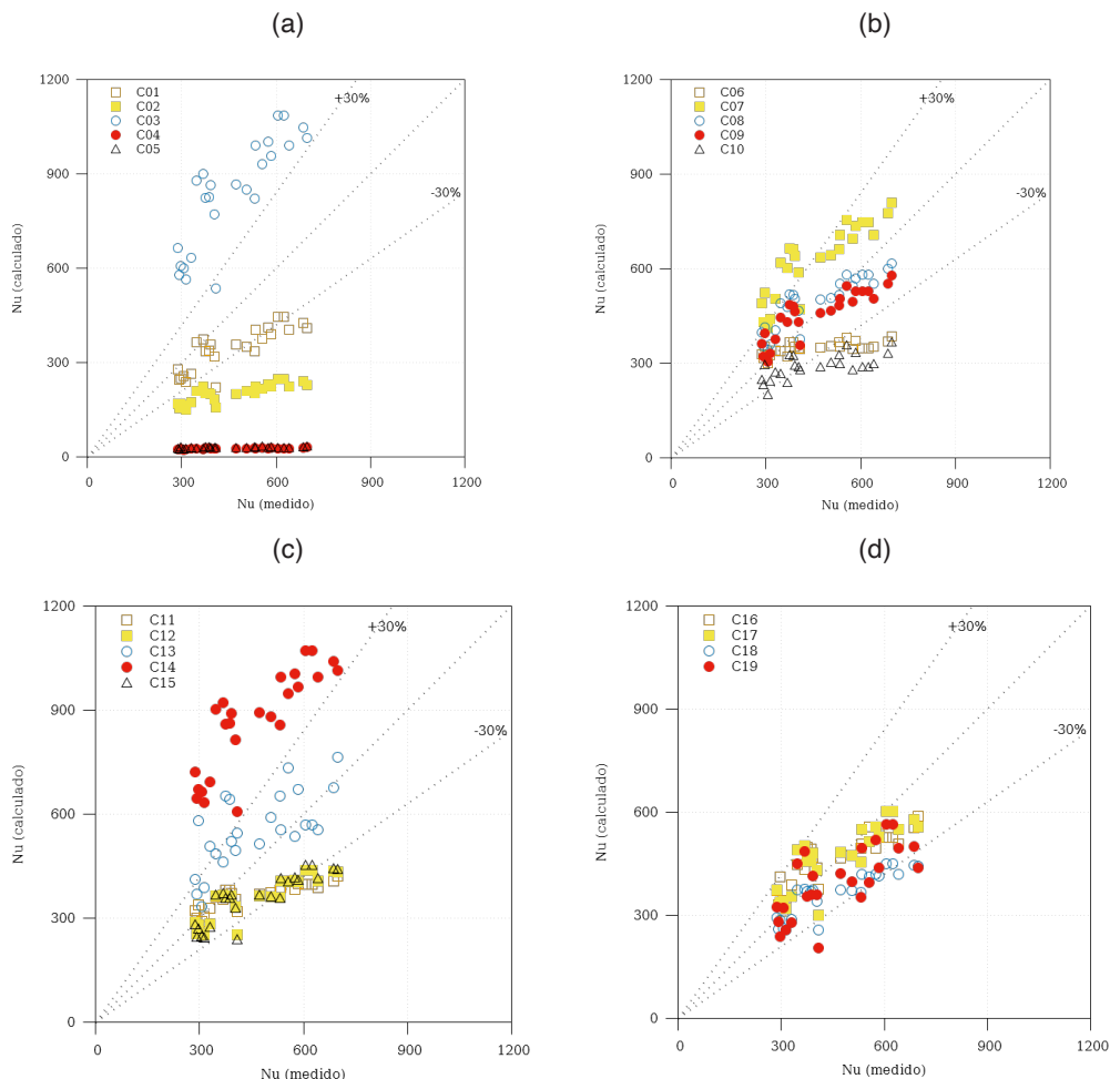
Figura 1 – Comparação dos resultados calculados e medidos, em termos do : (a) C01 a C05; (b) C06 a C10; (c) C11 a C15; (d) C16 a C19
