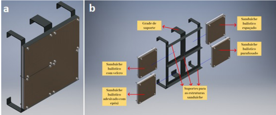
Figura 14: (a) conceito da estrutura completa; (b) componentes da estrutura completa.
