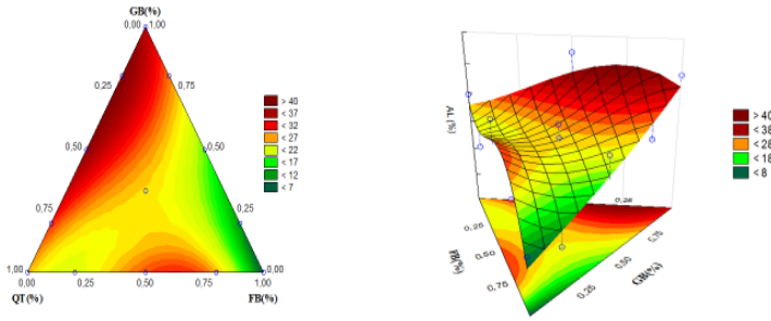
Figura 1: Superfícies de resposta para (a) Limite de Resistência à Tração (LRT), (b) Módulo de Elasticidade (ME) e (c) Alongamento na Ruptura (AI) dos filmes como função da concentração da fécula de batata, gelatina bovina e quitosana.
