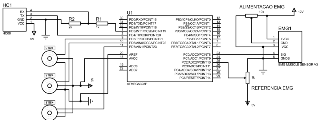
Figura 7 – Diagrama esquemático do circuito.
