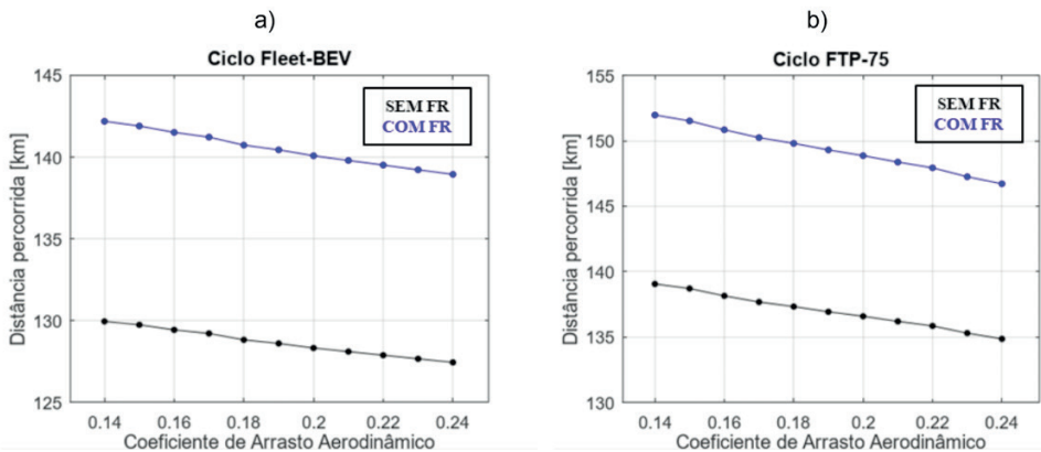
Figura 7 – Autonomia em relação ao coeficiente de arrasto aerodinâmico nos ciclos A e B
