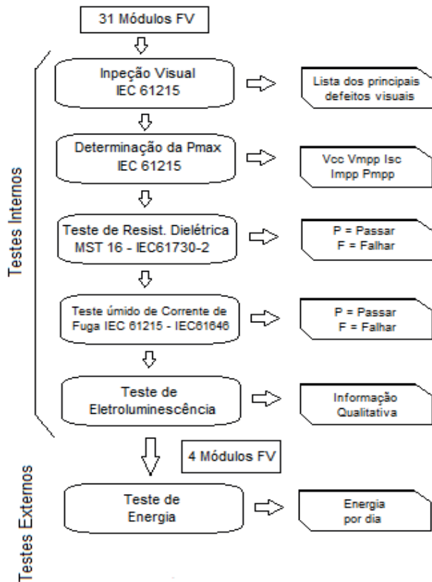
Figura 3 – Fluxograma de procedimento experimental
