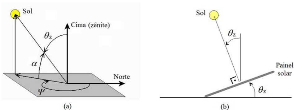
Figura 3 - (a) Ângulos solares \psi (Ângulo de azimute), \alpha (altitude solar) e \theta_z (ângulo de zênite); (b) Inclinação do painel solar para incidência normal dos raios solares.
