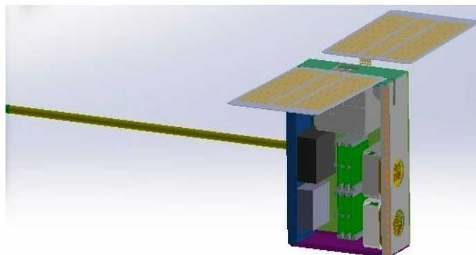
Figura 3 – CubeSat 6U em Ambiente CAD
