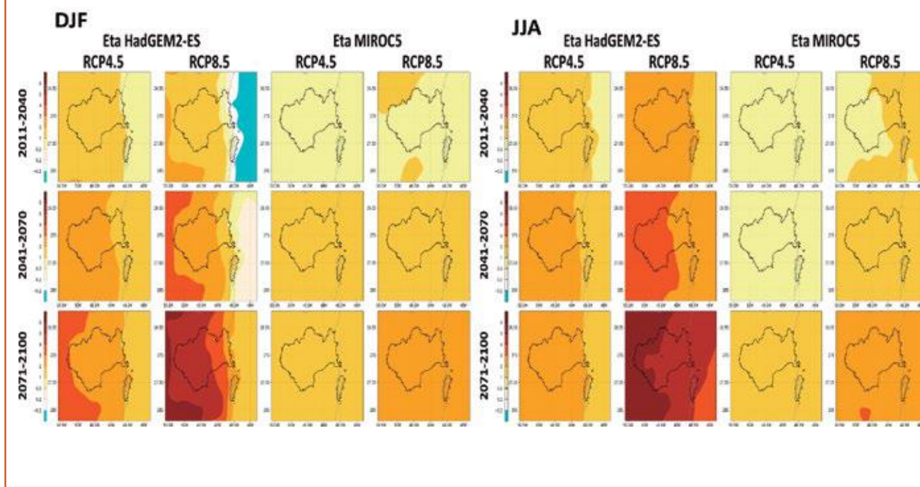
Figura 7.48 Projeções de temperatura do ar para DJF e JJA para a região do Vale do Itajaí. Projeções para 2011-40, 2041-70 e 2071-2100 são relativas ao presente (1961-90), para os cenários RCP 4,5 e 8,5, derivados do downscaling dos modelos HadGEM2-ES e MIROC5 usando o modelo regional Eta.
