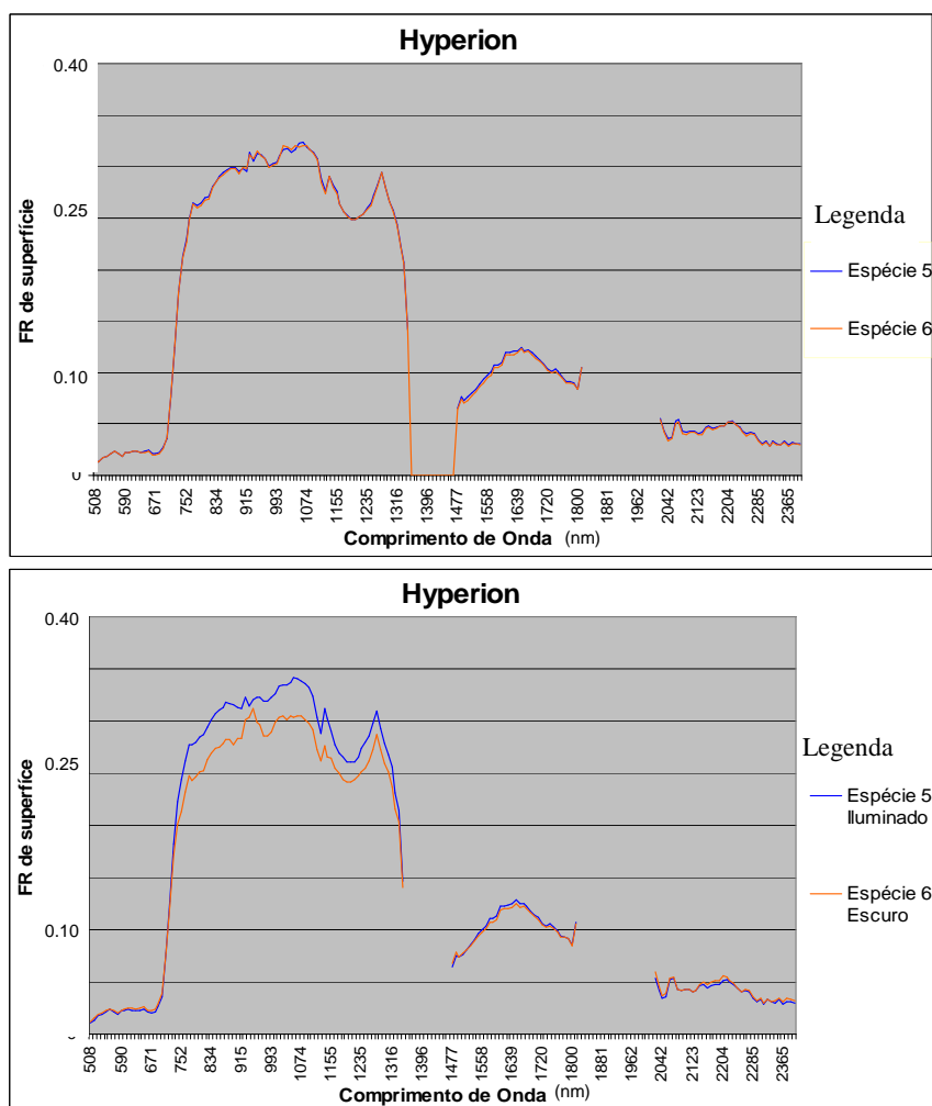
Figura 3. Comparação entre os espectros médios para espécies sem considerar a iluminação (acima) e os espectros para duas diferentes classes de iluminação. Figure 3. Comparison between the spectra average for the species without considering the illumination (above) and the spectra for two different classes of illumination.
