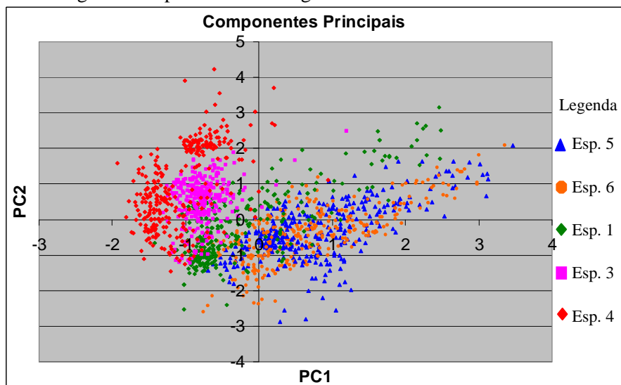
Figura 4. Primeiros dois fatores referentes às componentes principais 1 e 2 para as espécies de Eucalyptus spp. Figure 4. The first two factors for the principals components 1 and 2 for the species of Eucalyptus spp.
