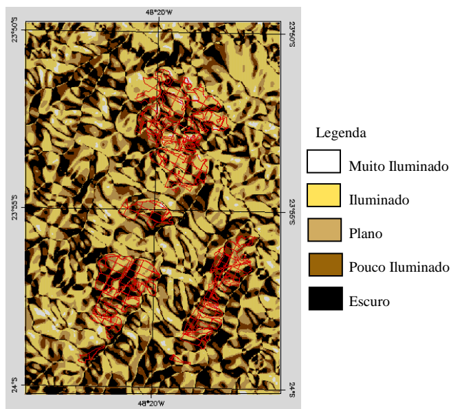
Figura 2. Classes de iluminação referentes à imagem de 2003. Figure 2. Illumination classes for 2003 image.
