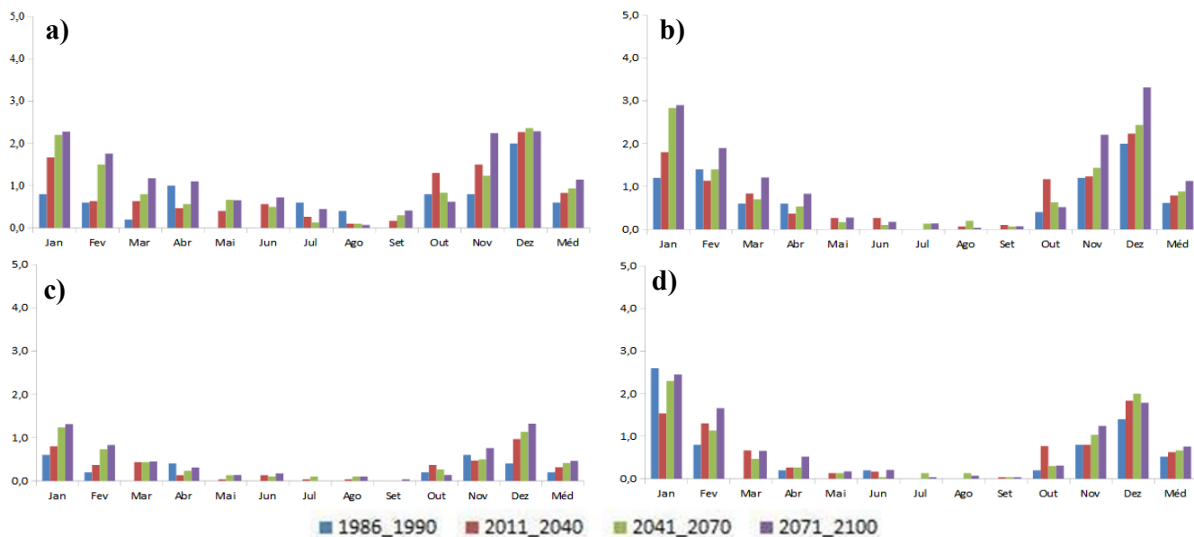
Figura 3 - Número de dias cuja precipitação ultrapassou 30 mm, segundo as simulações do modelo Eta/CPTEC para o clima presente (1986-1990) e projeções do cenário A1B (2011-2040; 2041-2070; 2071-2100), para as cidades de: a) Campinas, b) Mococa, c) Pindorama e d) Ribeirão Preto, localizadas no estado de São Paulo
