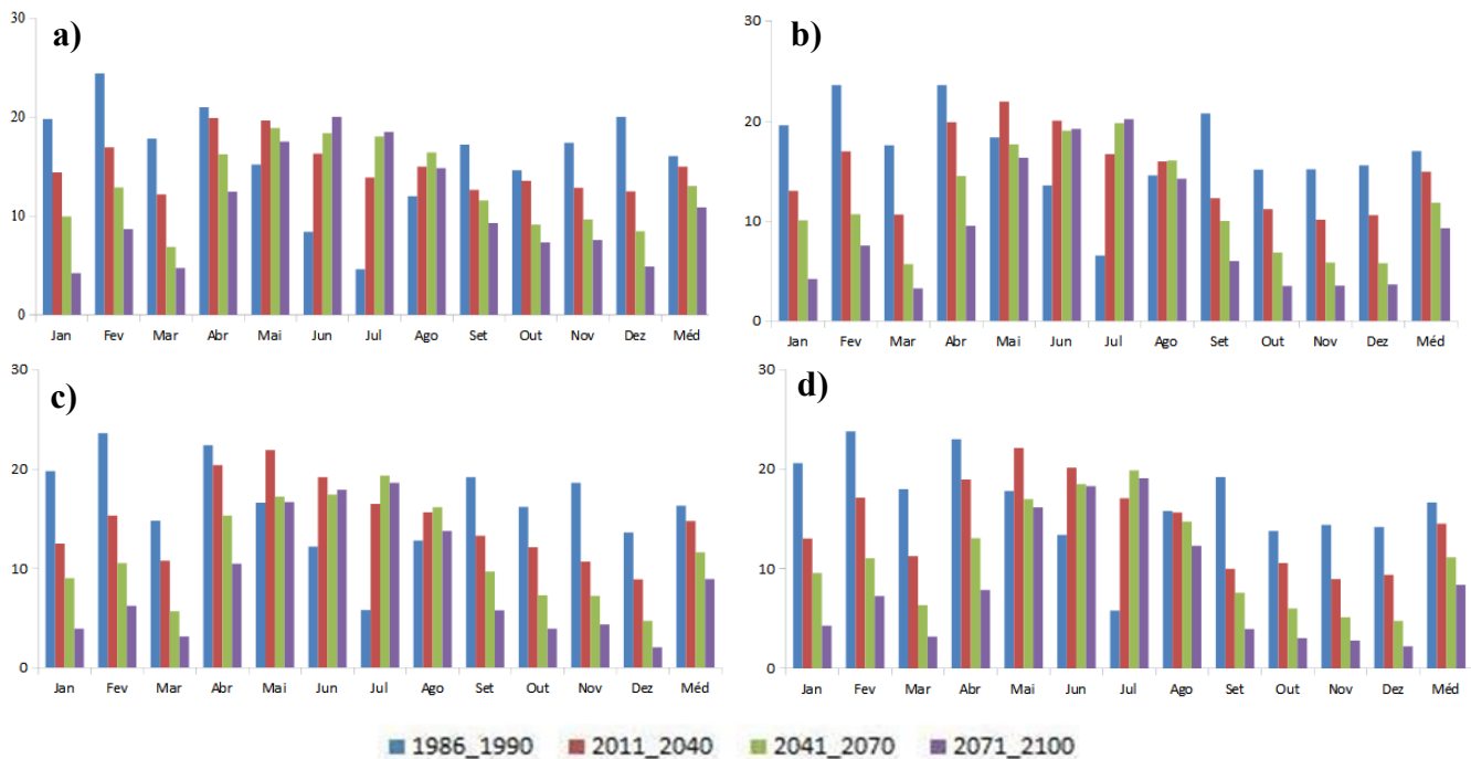
Figura 2 - Número de dias com temperatura média entre 20 e 25°C, segundo as simulações do modelo Eta/CPTEC para o clima presente (1986-1990) e projeções do cenário A1B (2011-2040; 2041-2070; 2071-2100), para as cidades de: a) Campinas, b) Mococa, c) Pindorama e d) Ribeirão Preto, localizadas no estado de São Paulo
