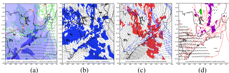
Figura 4: (a) Umidade relativa do ar média (URM) > 60% em 850-500 hPa (sombreado), URM em 1000-850 hPa (contorno) e vento > 5m/s; (b) omega < -2.10^{-5} \text{ s}^{-1} , URM (1000-850) e URM (850-500hPa) > 60% (sombreado), linha de corrente em 500 hPa ; (c) URM em 1000/850 hPa e 850/500 hPa > 60%; omega em 500 hPa < -2.10^{-5} \text{ s}^{-1} ; Total Totals > 45 e K > 30 (sombreado vermelho) e divergência em 250 hPa (contorno azul); (d) idem c, mas com (TTS) > 48, K > 33.
