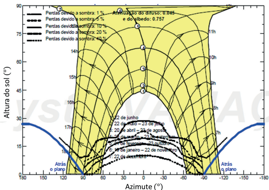
Figura 1: Análise de sombreamento - software PVsyst
