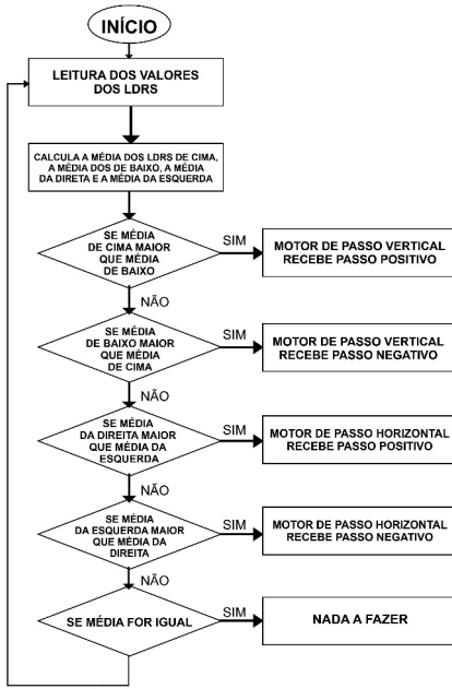
Figura 6 – Pseudocódigos para os seguidores solares.
