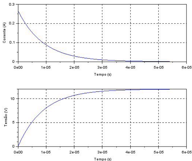
Figura 4. Resultado computacional para o circuito RL.
