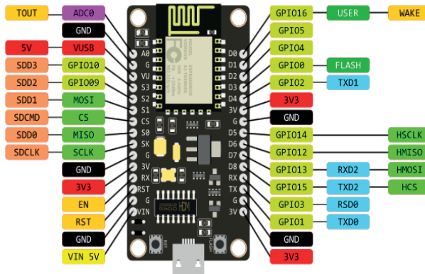
Figura 5- Pinagem de nodemcu.
