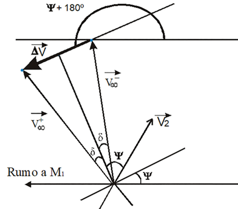
Figura 3: Vetores velocidade envolvidos em uma manobra de swing-by .
